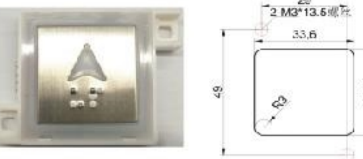
MR-EPB013-F
